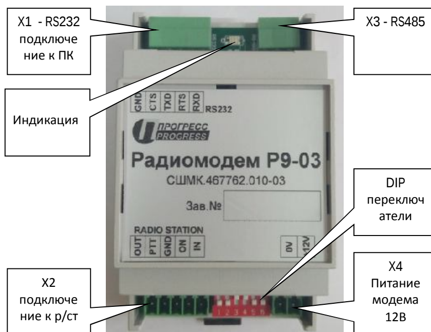
Рис. 2 Расположение разъемов и переключателей
